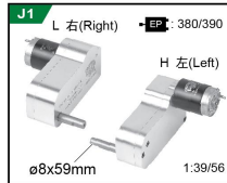
J1 CNC驱动波箱(“匠”系列) CNC drive gear box (“Craftsman”series)
